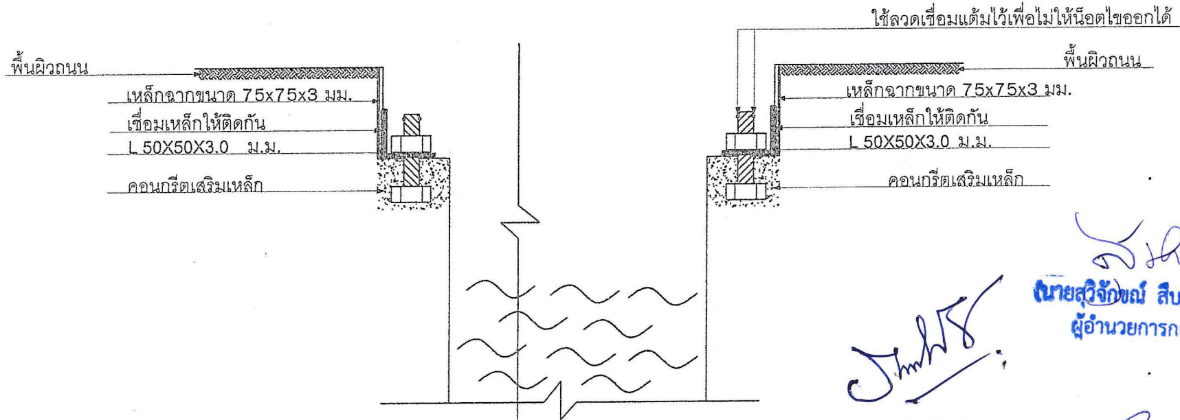
แบบขยายการติดตั้งน๊อตทุก ไม่กำหนดมาตราส่วน
