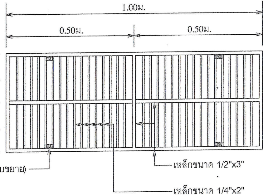
แบบขยายฝาร่างระบายน้ำ ไม่กำหนดมาตราส่วน
