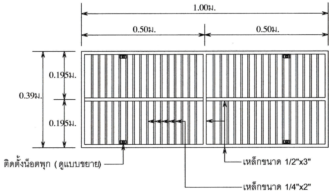
แบบขยายฝารางระบายน้ำ
